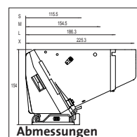
Abmessungen
